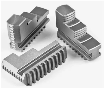
Прямые кулачки для токарных патронов серии 7100
